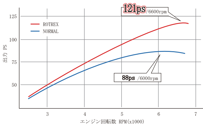
出力比較グラフ
