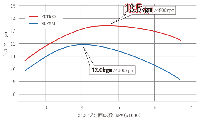
トルク比較グラフ
